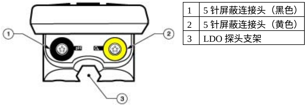
图 3 探头连接器
