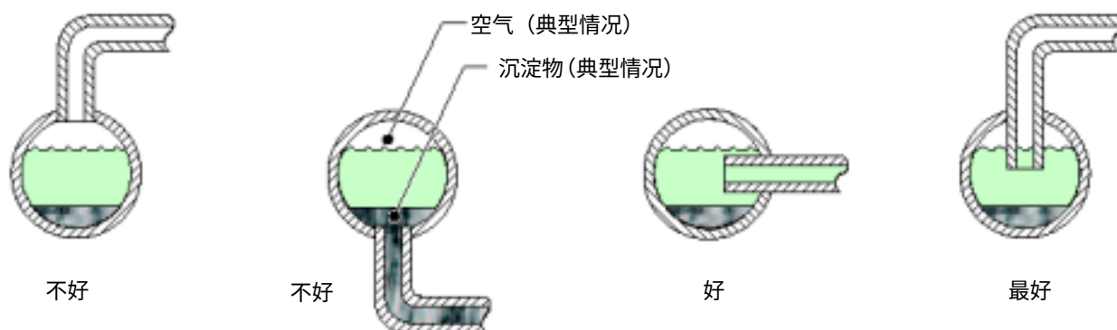
图 24 取样技术
